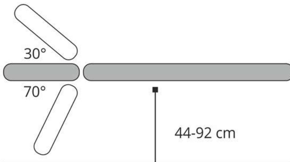
Pozycjonowanie blatu
