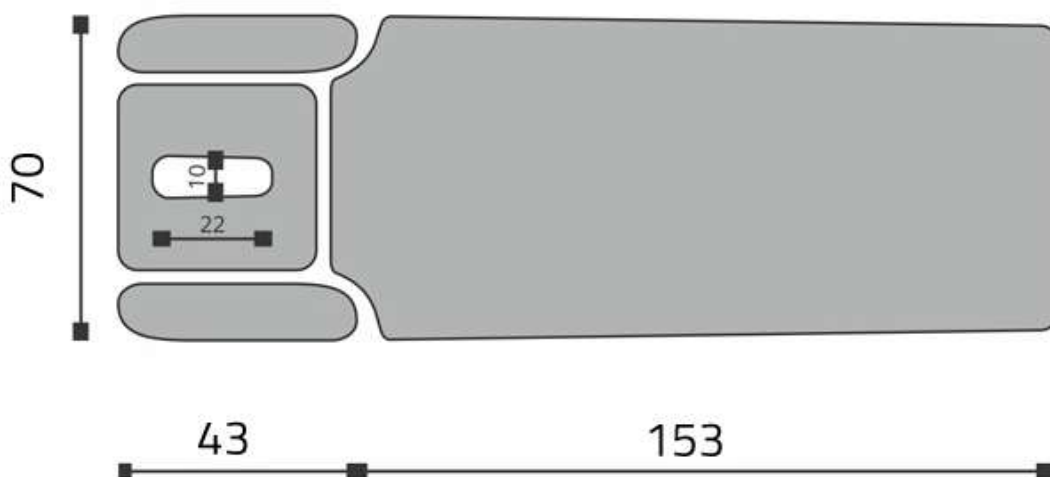
Wymiary blatu
