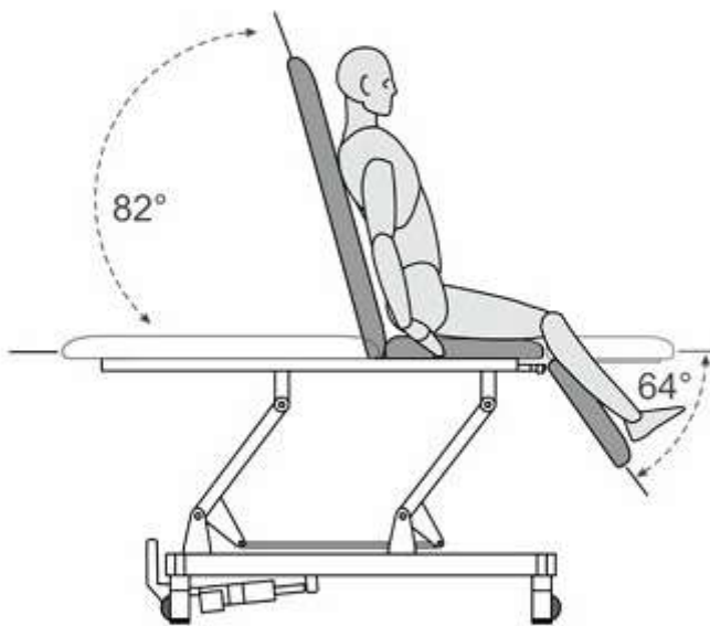
Pozycjonowanie blatu
